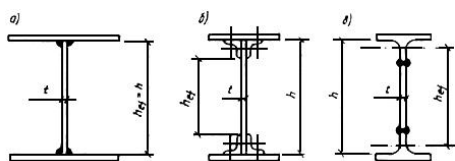
Рис.10. Расчетная высота стенки составной балки
