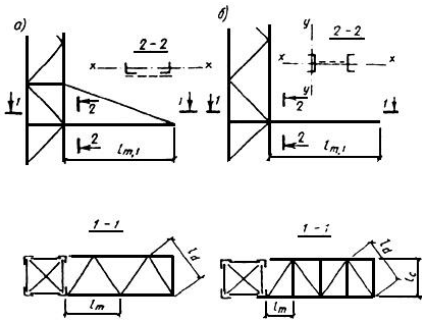
Рис.21. Схемы траверс
