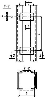
Рис.3. Составной стержень на планках
