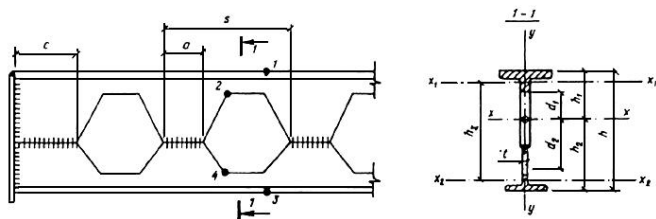
Рис.23. Схема участка балки с перфорированной стенкой
