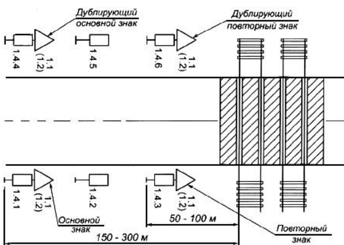
Рисунок В.3 - Размещение знаков 1.4.1-1.4.6
