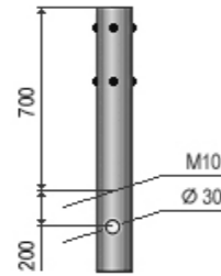
Воздушный подвод кабеля Верхняя часть опоры
