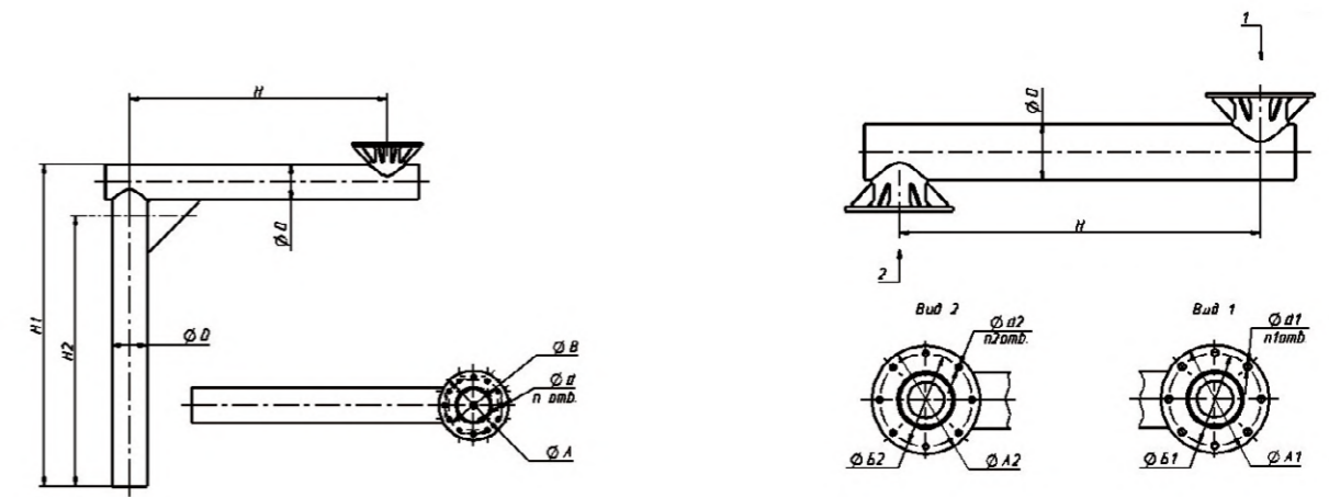
Консольная закладная деталь
